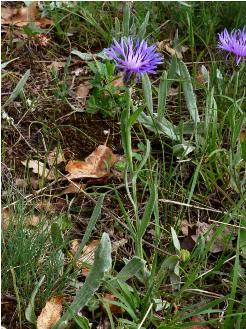
Centaurea triumfettii
